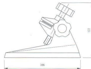
MICROMETER STAND
