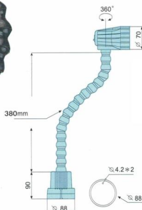
VHL-600FT
