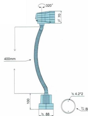
VHL-700FT
