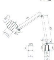
VHL-400L
