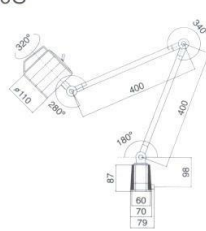
VHL-500L
