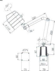
VHL-400M
